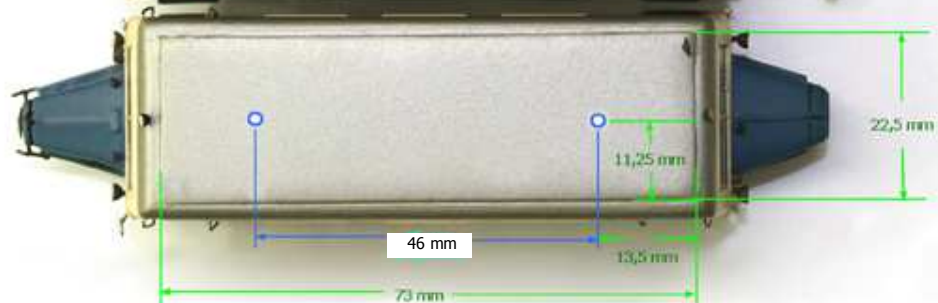
Dachpartie nach Umbau mit neuem Dacheinsatz
