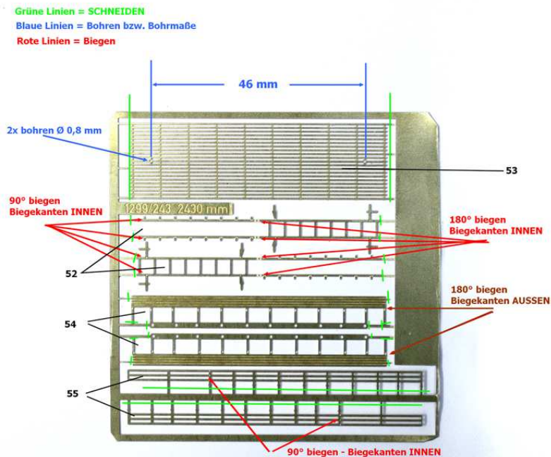
Dachpartie des Heinzl-Merker&Fischer-Bemo-Gehäuses
